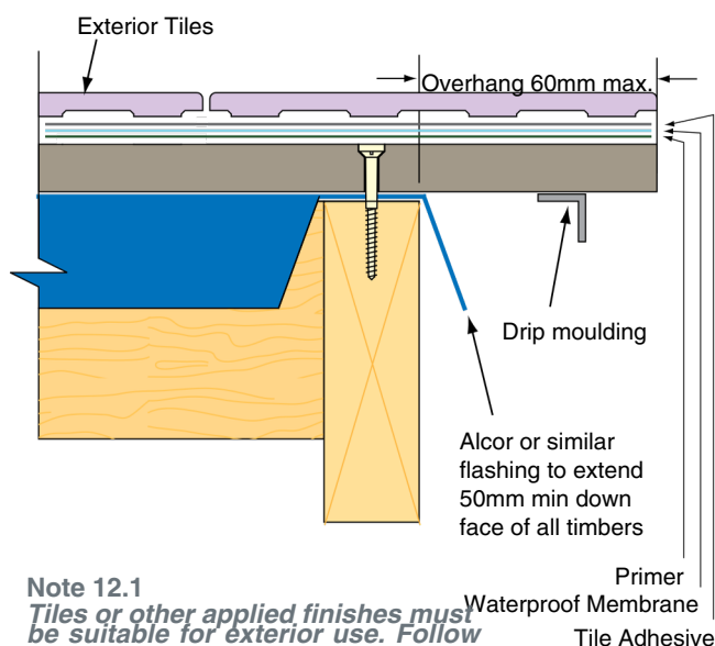
FIGURE 12 // EDGE DETAIL
