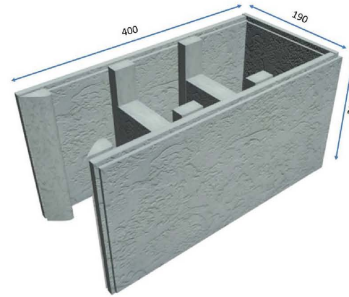
VERSALOC END BLOCK
