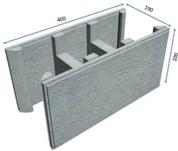
VERSALOC STANDARD BLOCK
